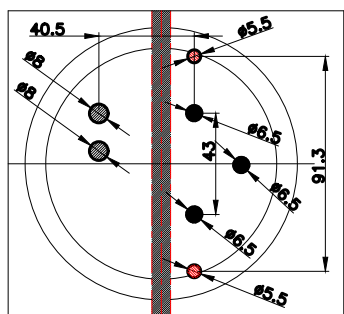
Bore skabelon
